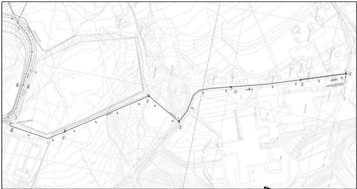
Figur 30 Eksisterende VA, forsterket vannforsyning fra Elvegårdsmoen, Multiconsult
