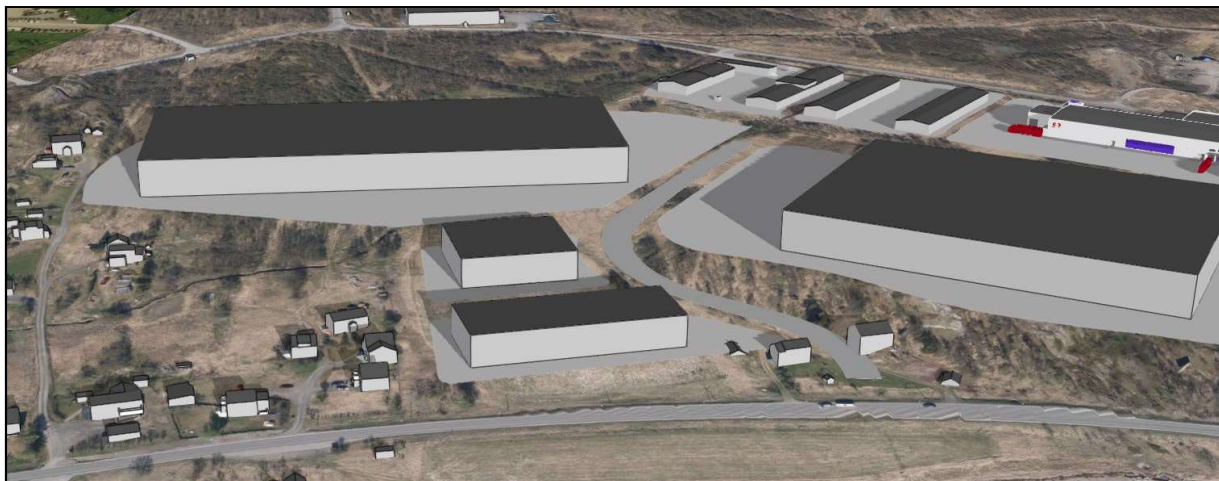
Figur 42 Solforhold 15/3 kl. 15 for alt. H1, næringsbebyggelsen skygger kun egen tomt
